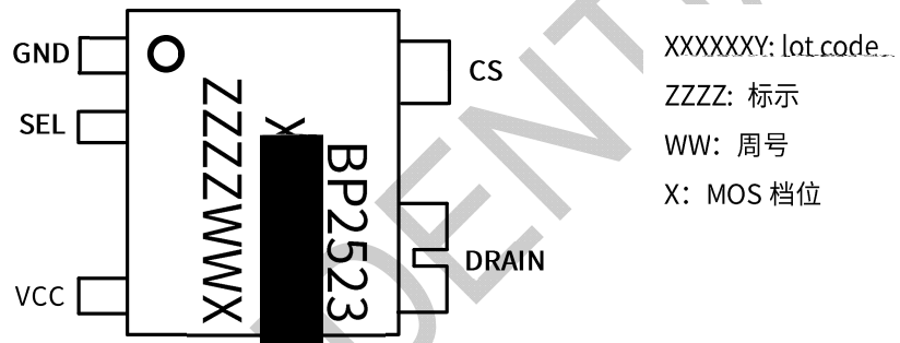
图 2 管脚封装图
